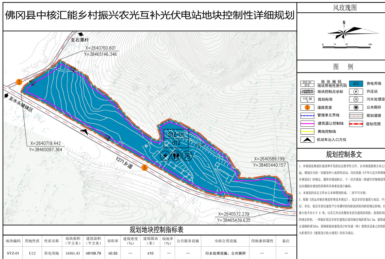
图 2 用地规划图
