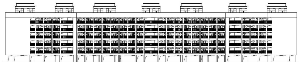
③-③剖面图 151
