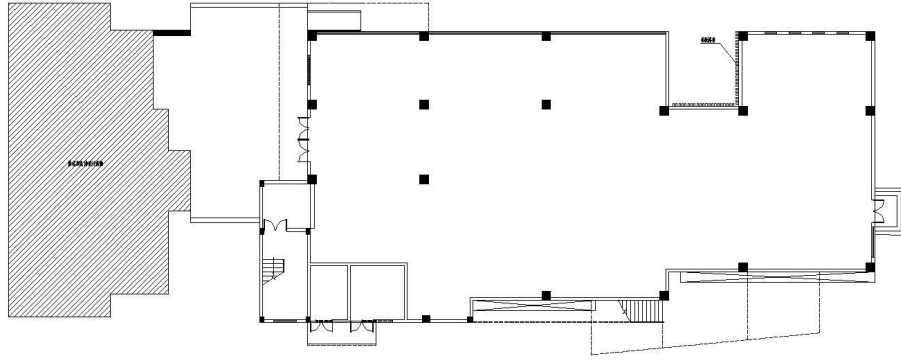
一层平面图 1:100
