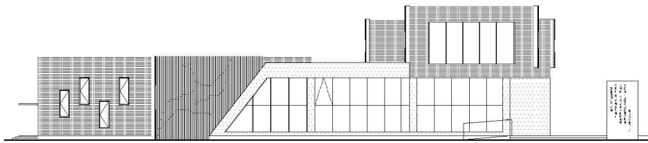
⑩-⑩轴立面图 1:150
