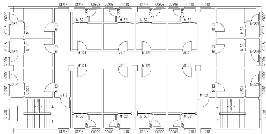
二层平面图 1:100
