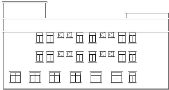
① ⑥轴立面图 1:100
