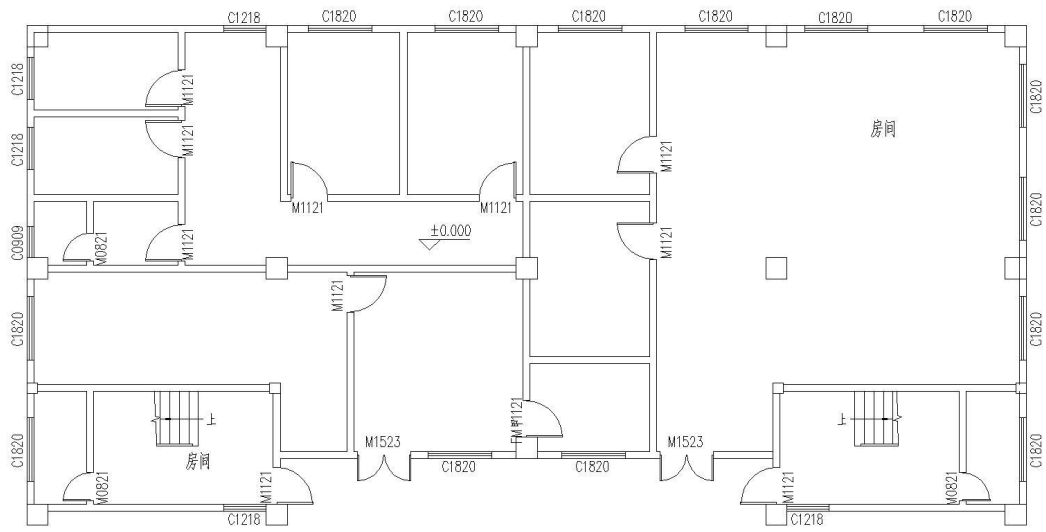
首层平面图 1:100
