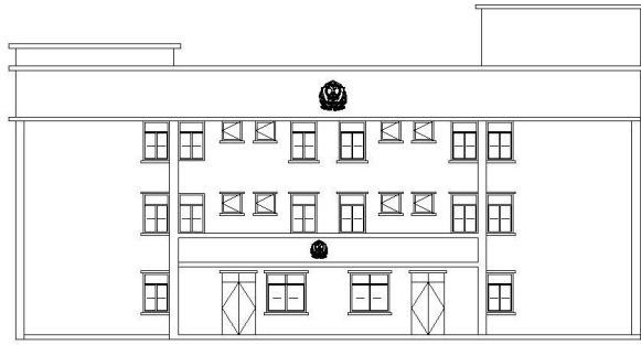
① ⑥轴立面图 1:100
