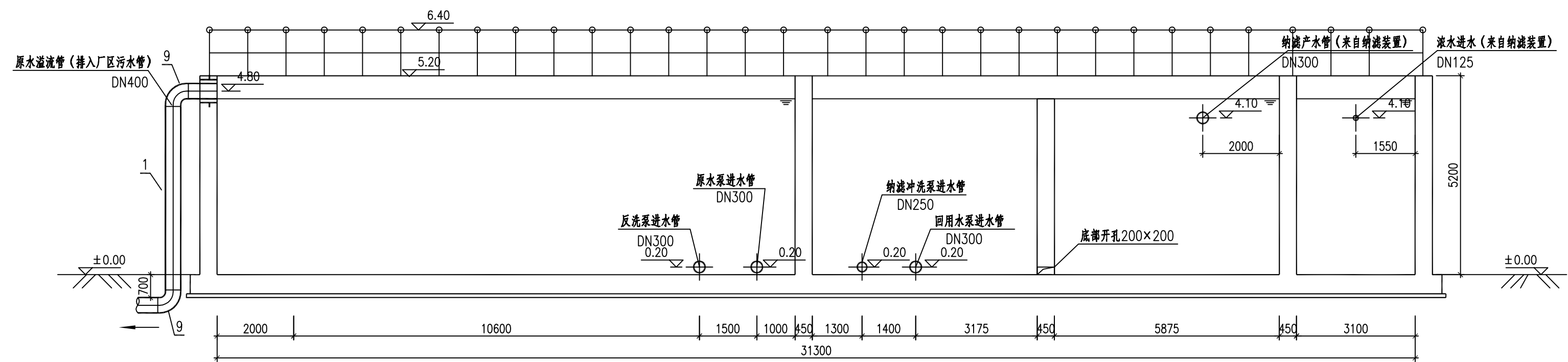
2-2剖面图 1:100
