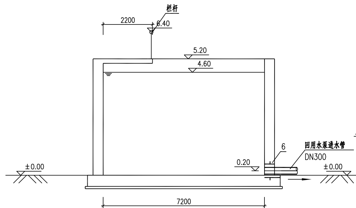
4-4剖面图 1:100
