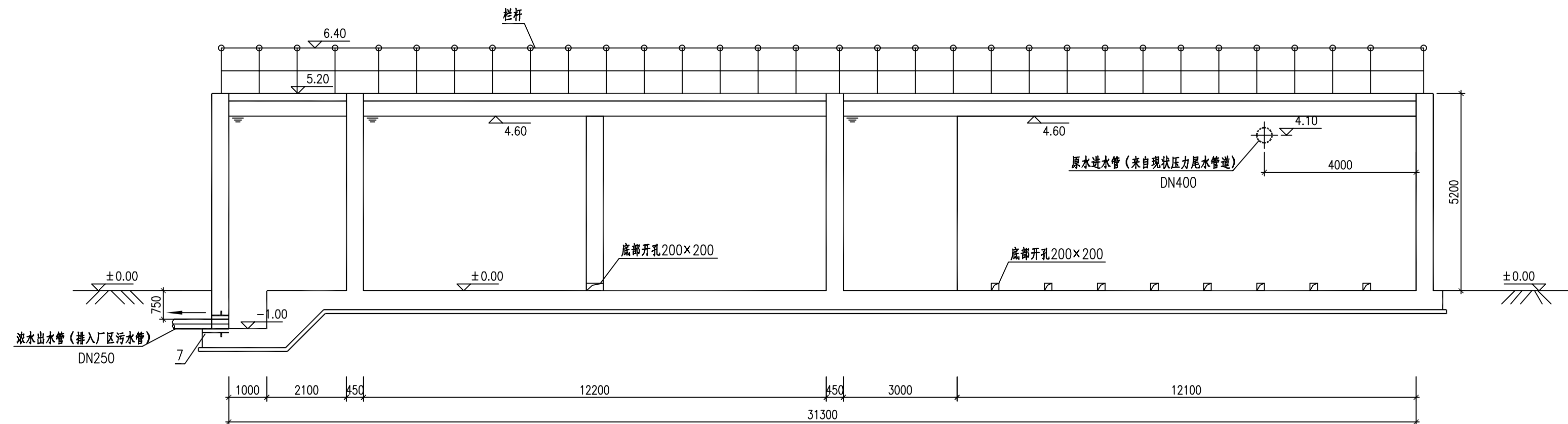
1-1剖面图 1:100
