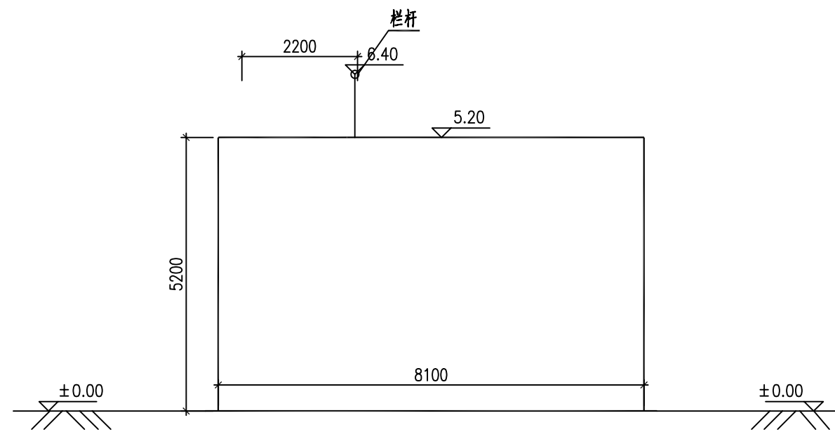
侧立面图
