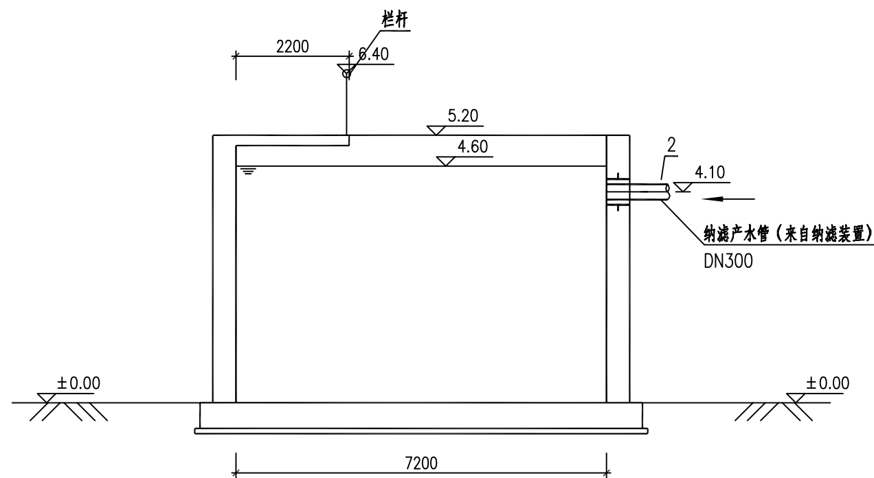
3-3剖面图 1:100
