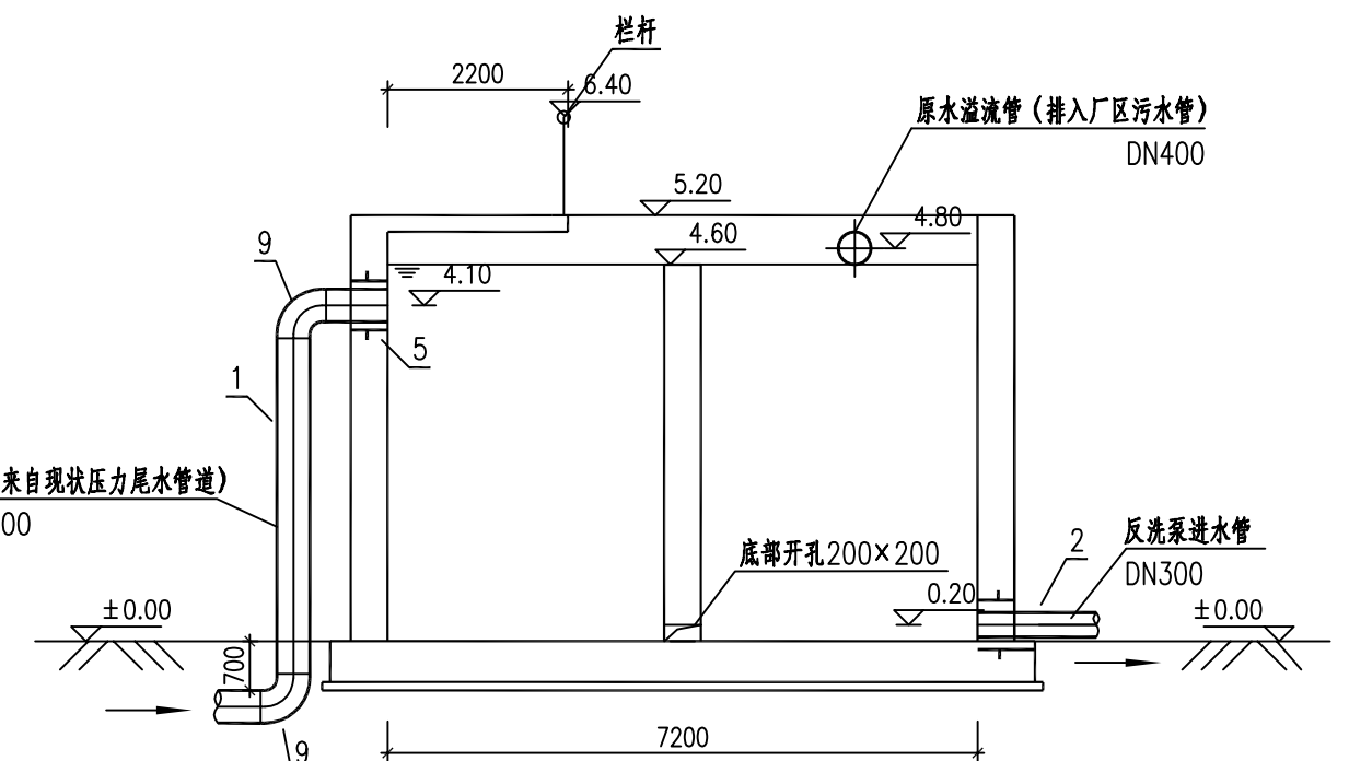
5-5剖面图 1:100
