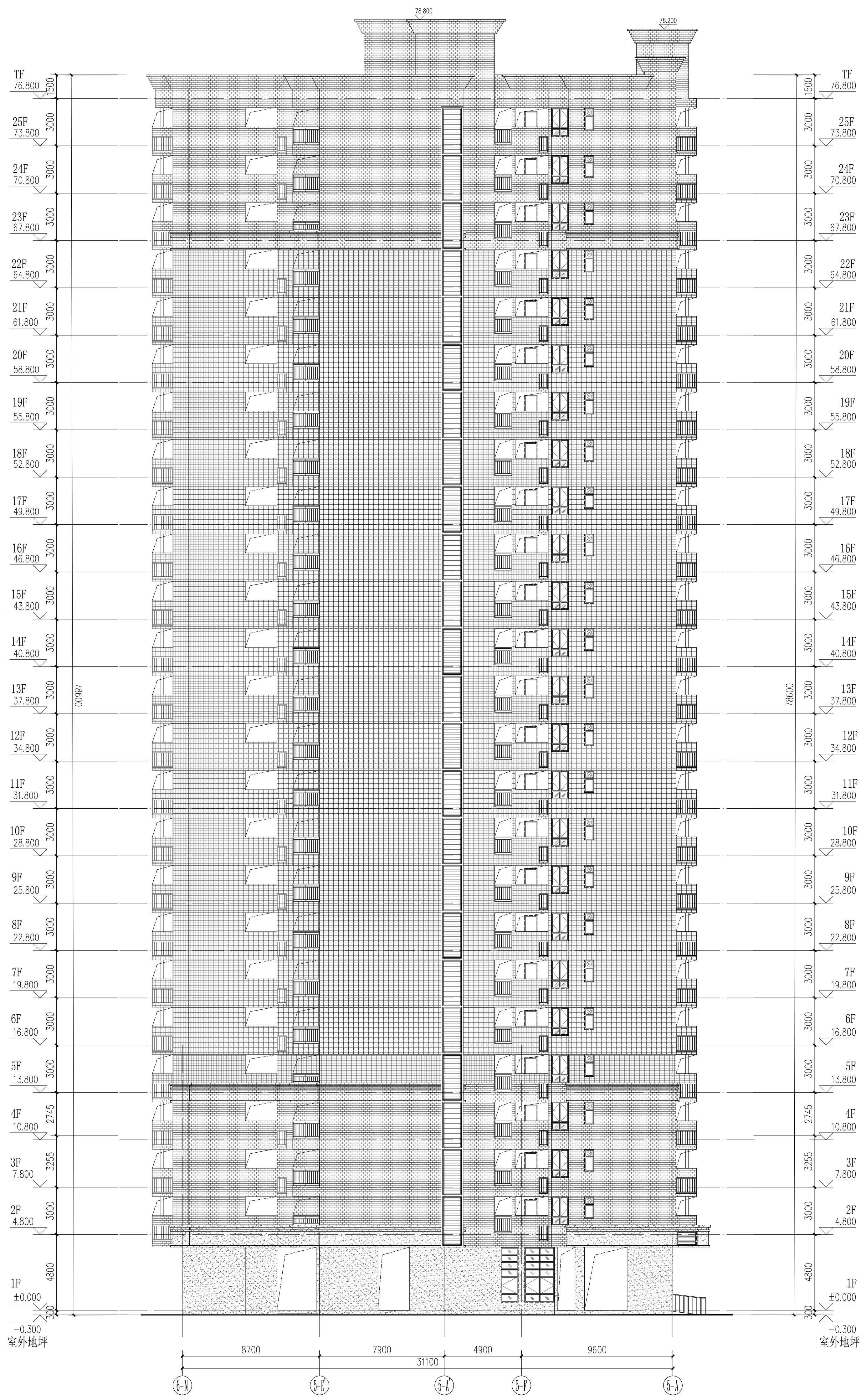
⑥-⑩轴立面图 1:150
