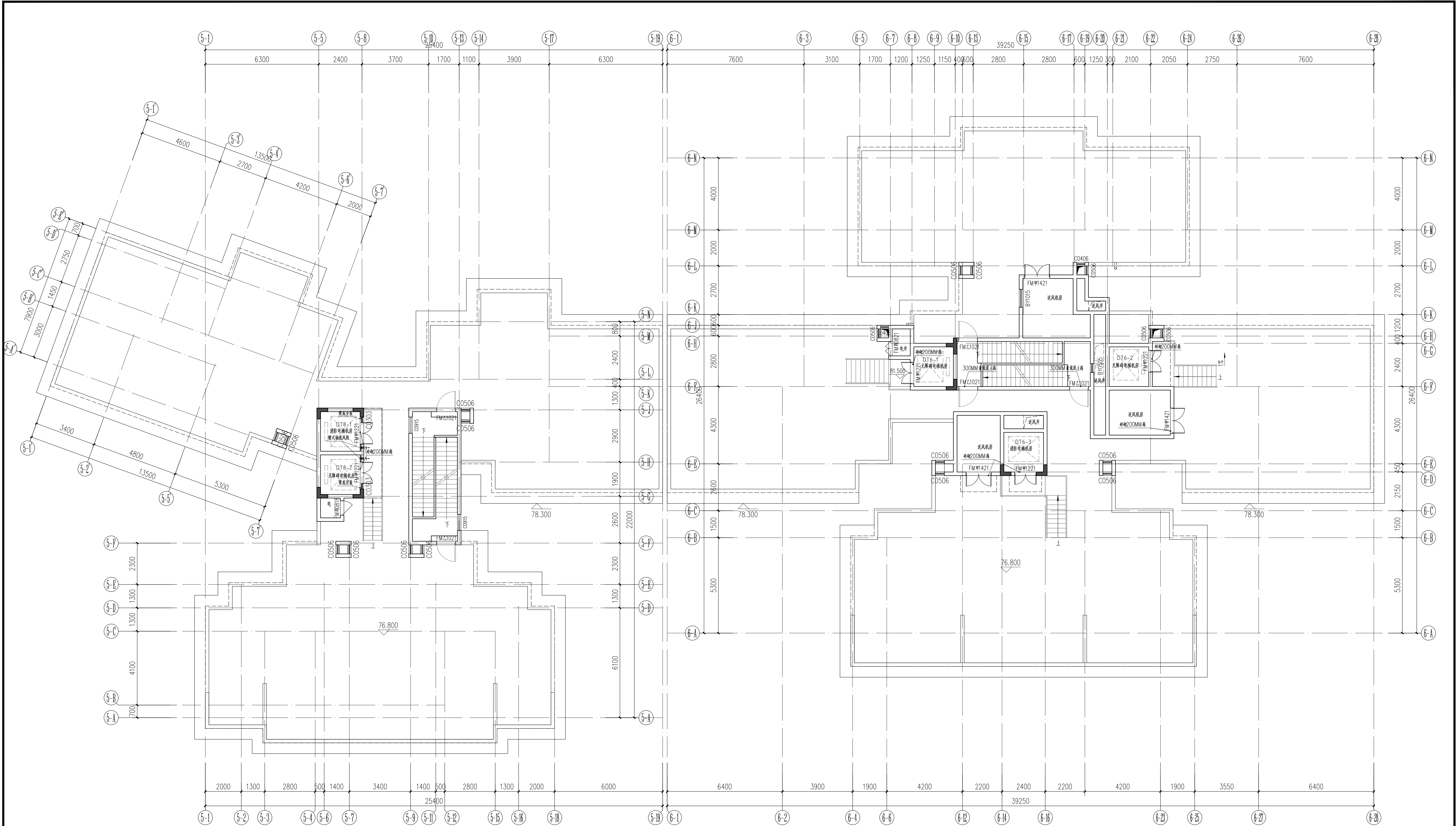
屋面层平面图 1:100
