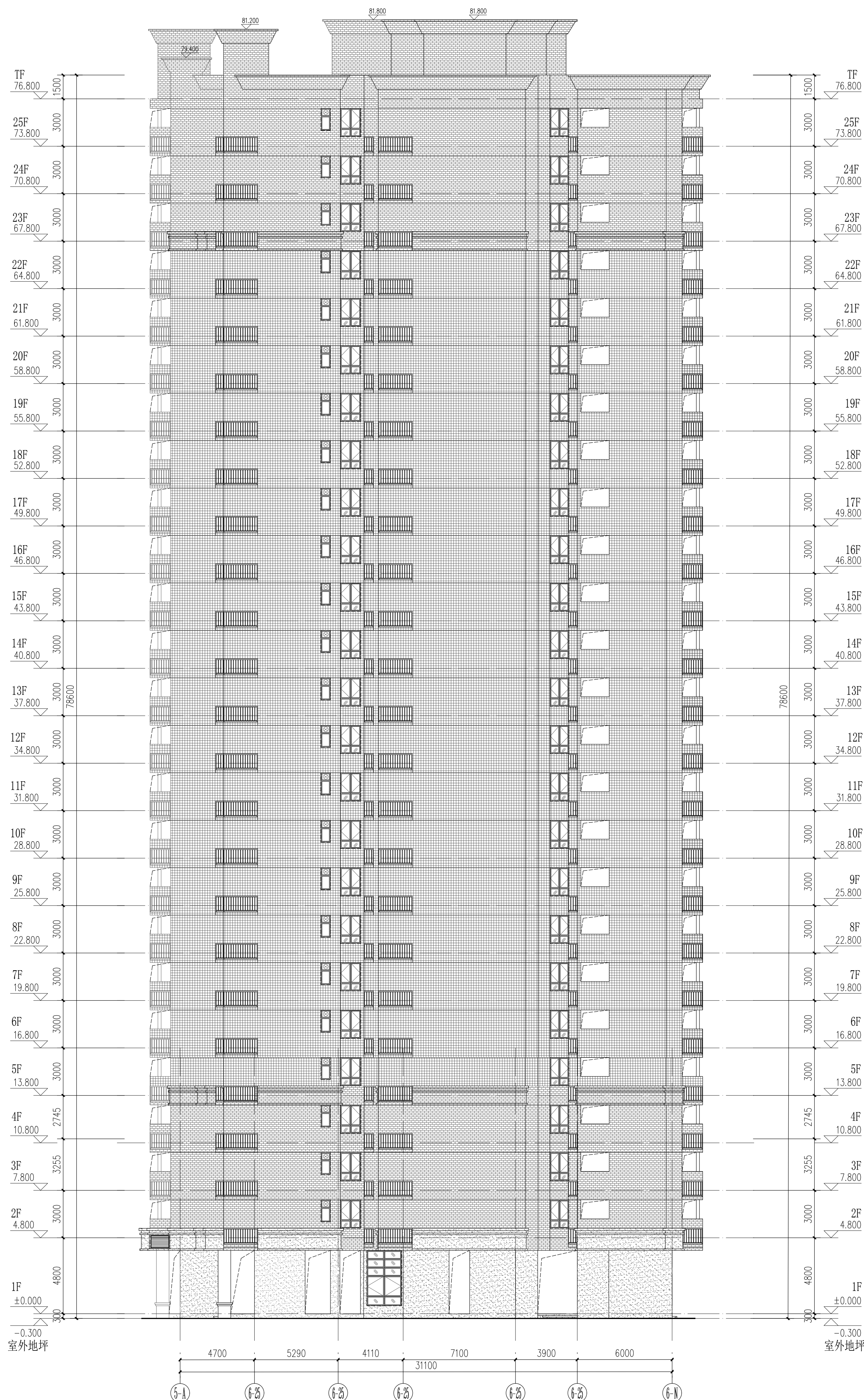
⑤-①~⑤-②③轴立面图 1:150
