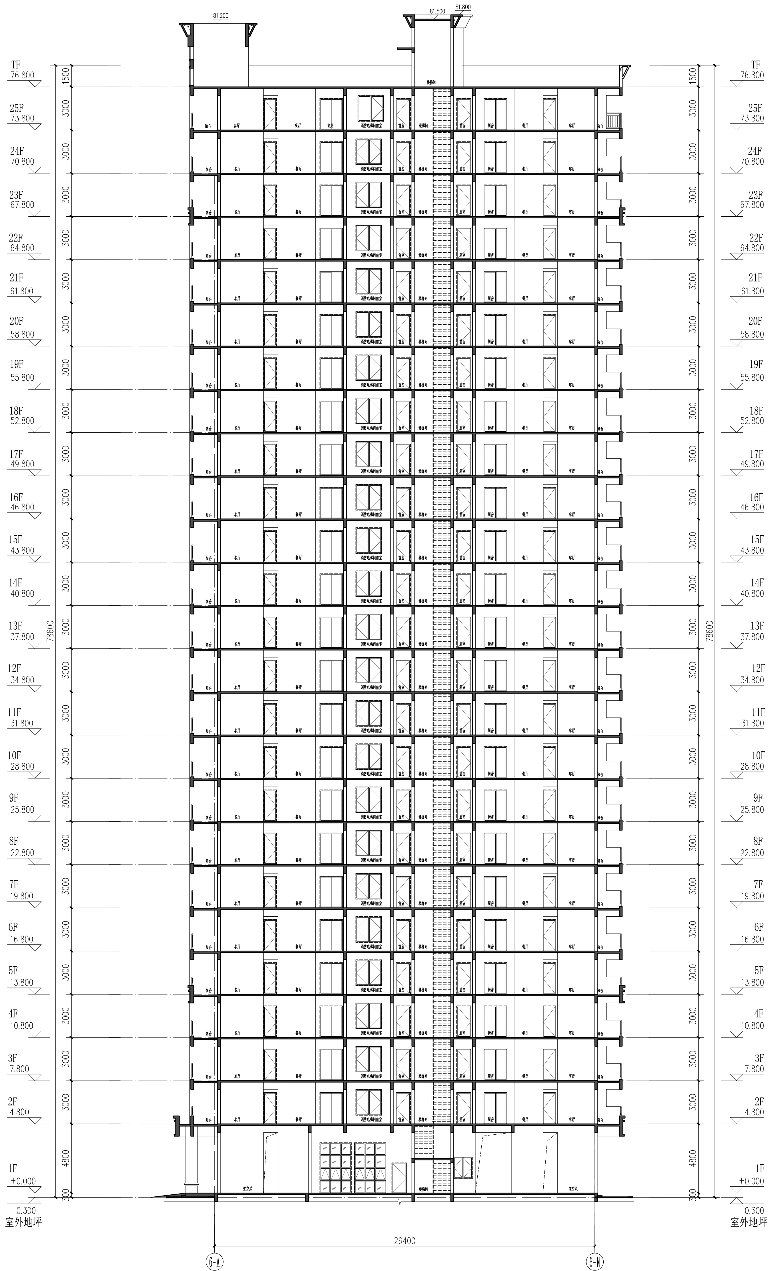
1-1剖面图 1 : 1 5 0
