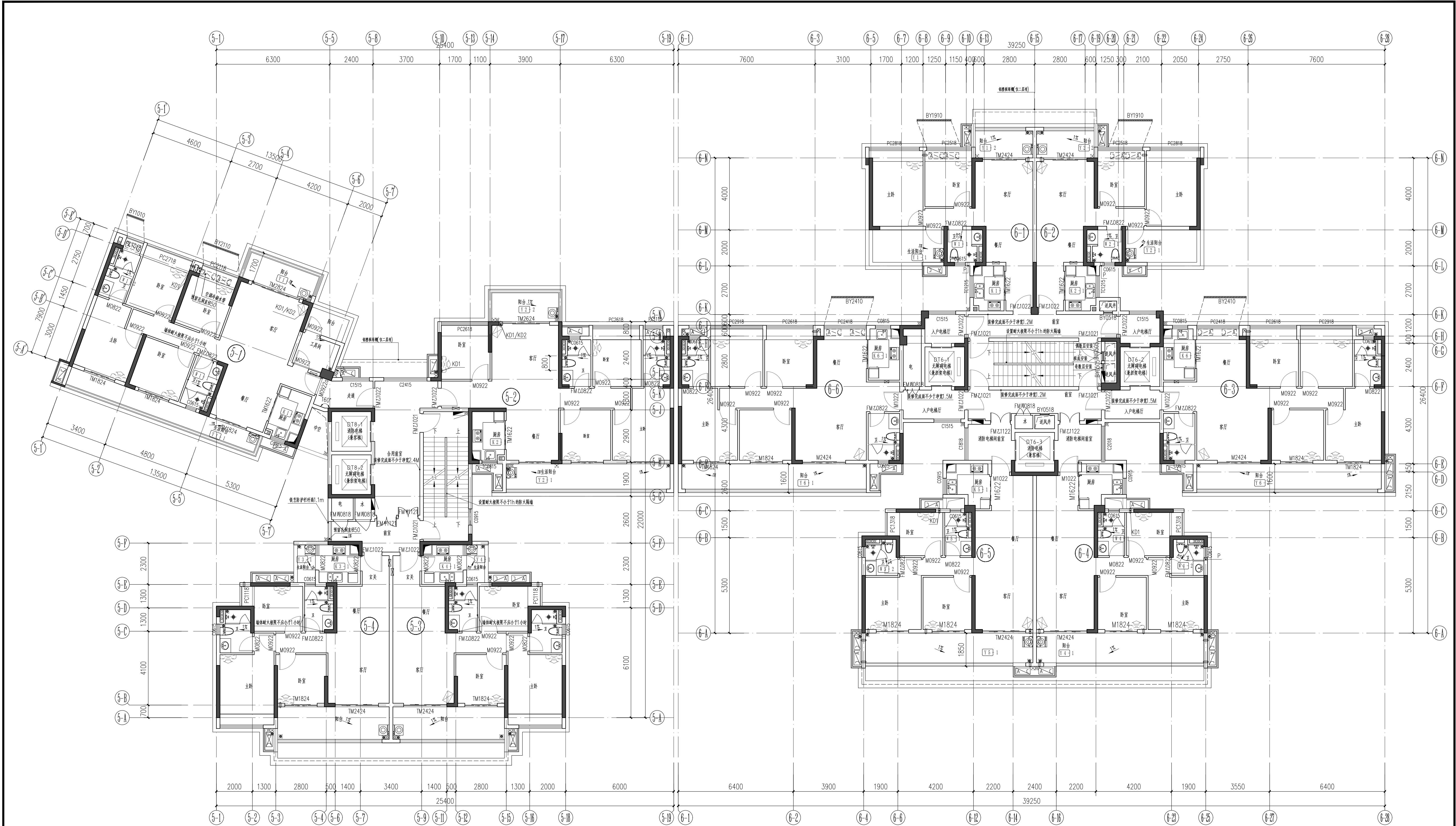
二层平面图 1:100
