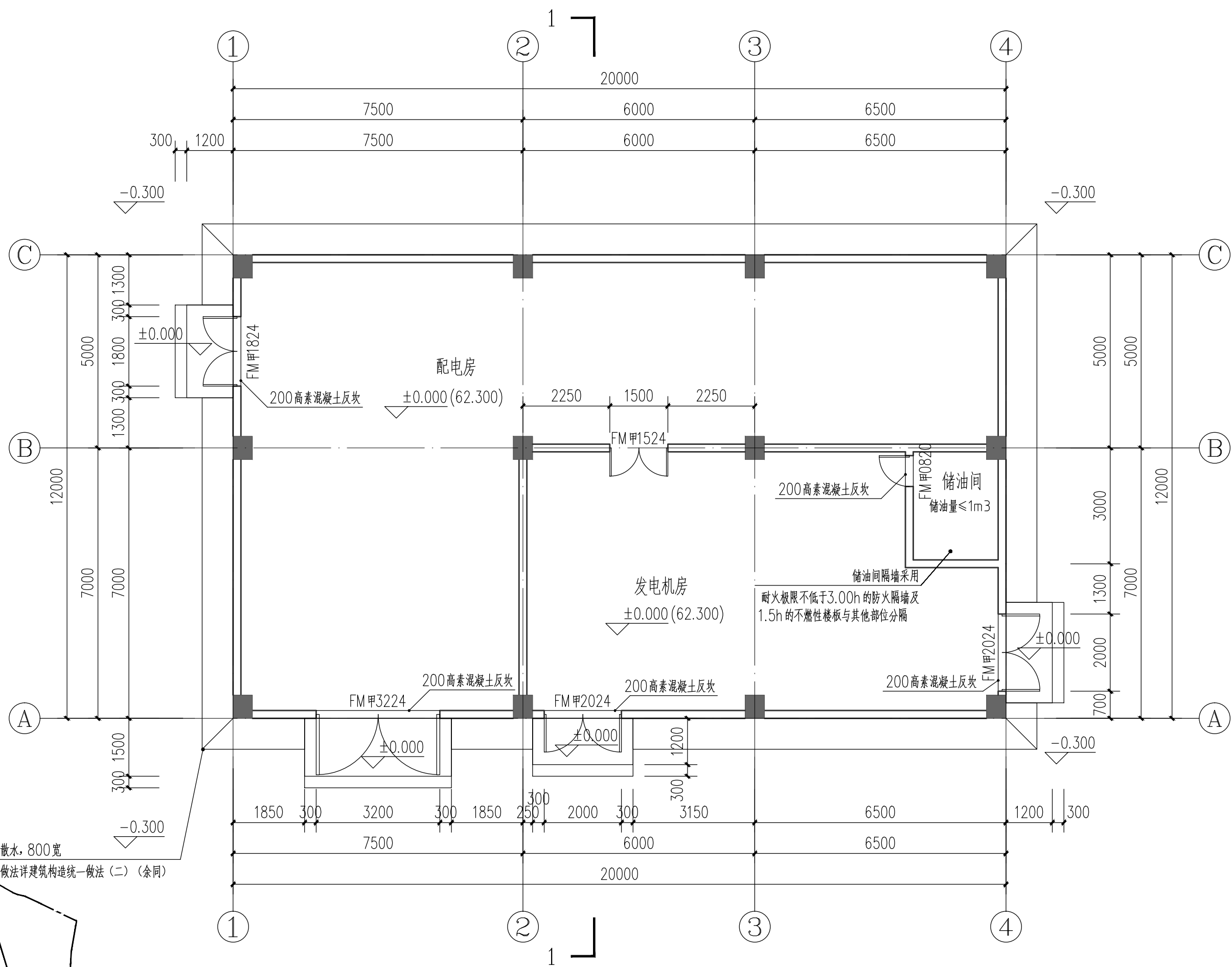
首层平面图 1:100
