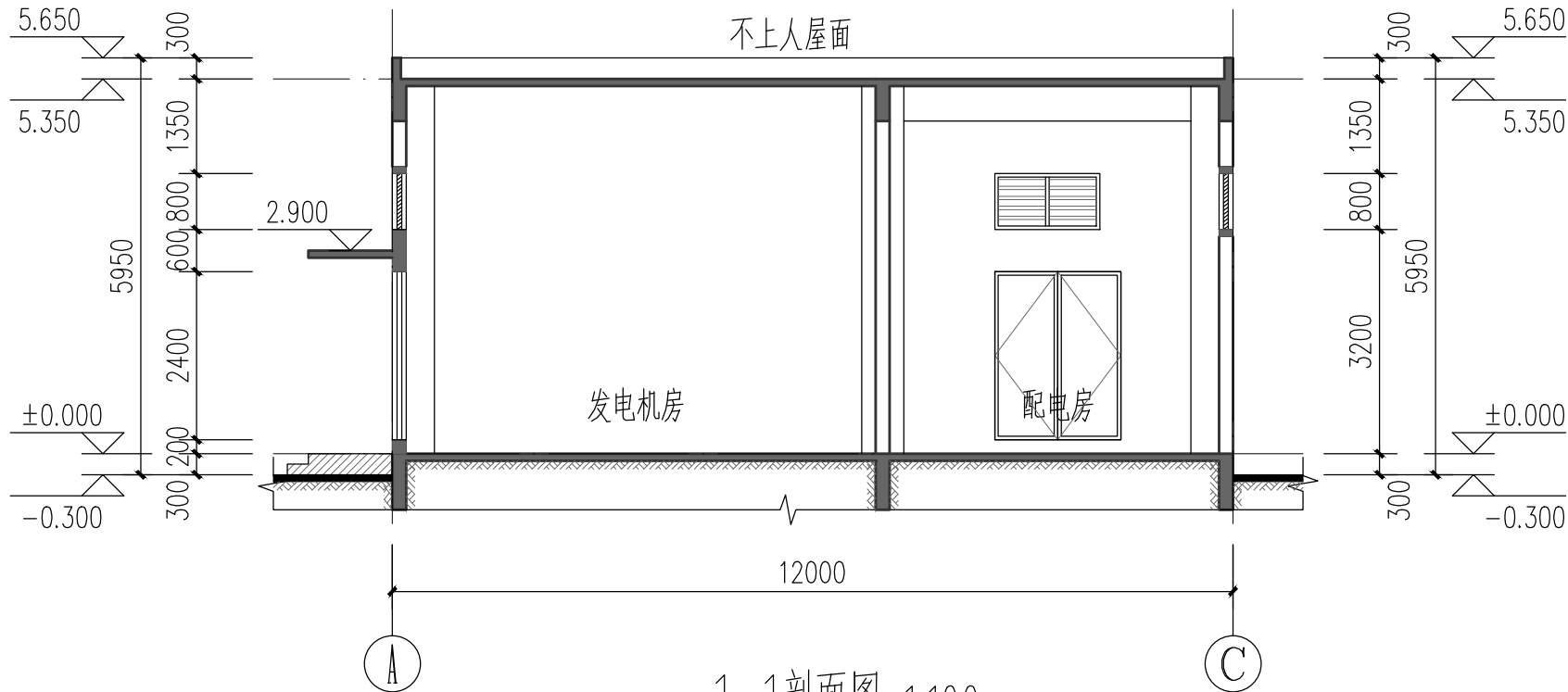
1-1剖面图 1:100
