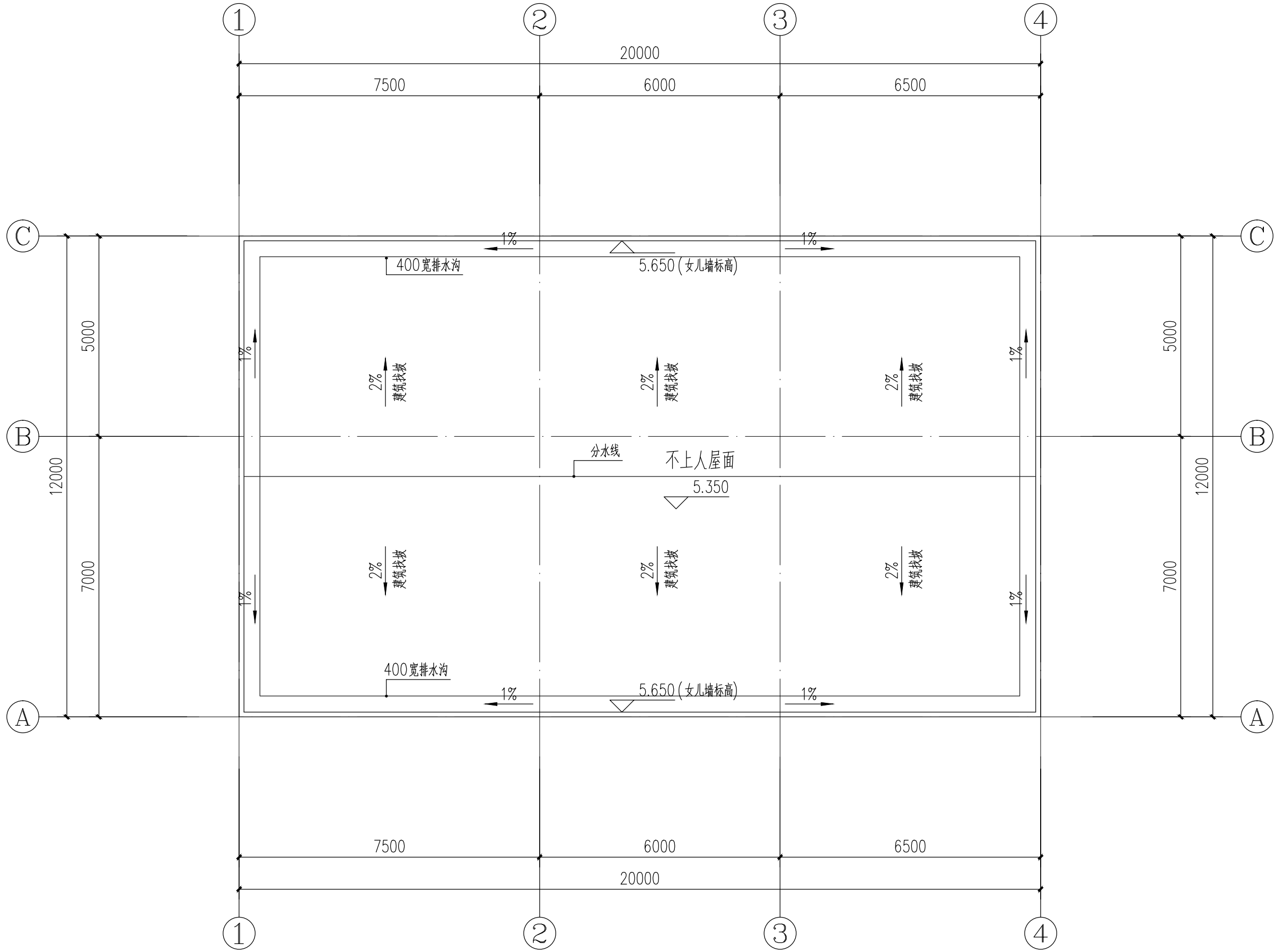
屋面层平面图 1:100
