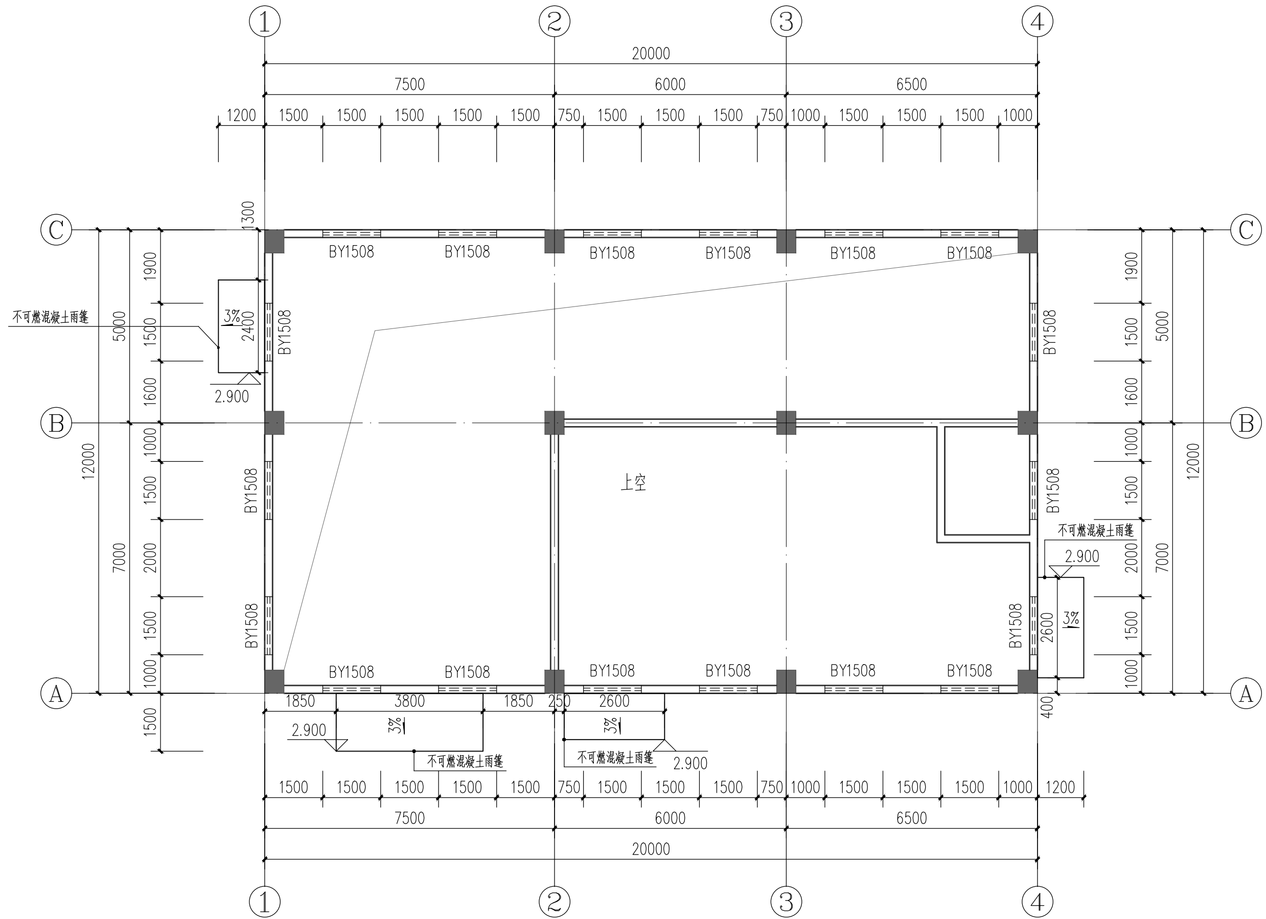
3.0m标高处平面图 1:100
