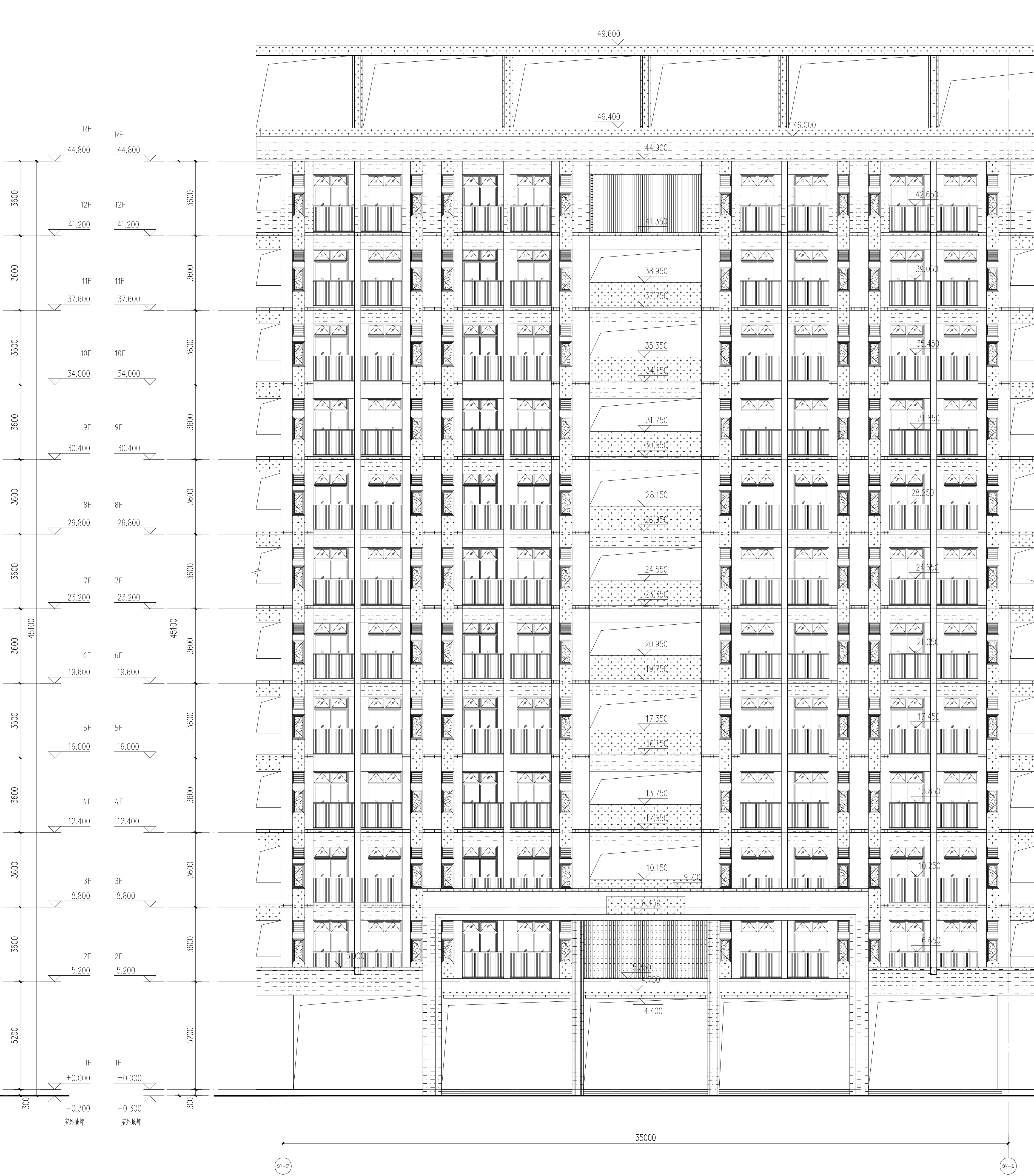
⑭~⑮立面图 1:100
