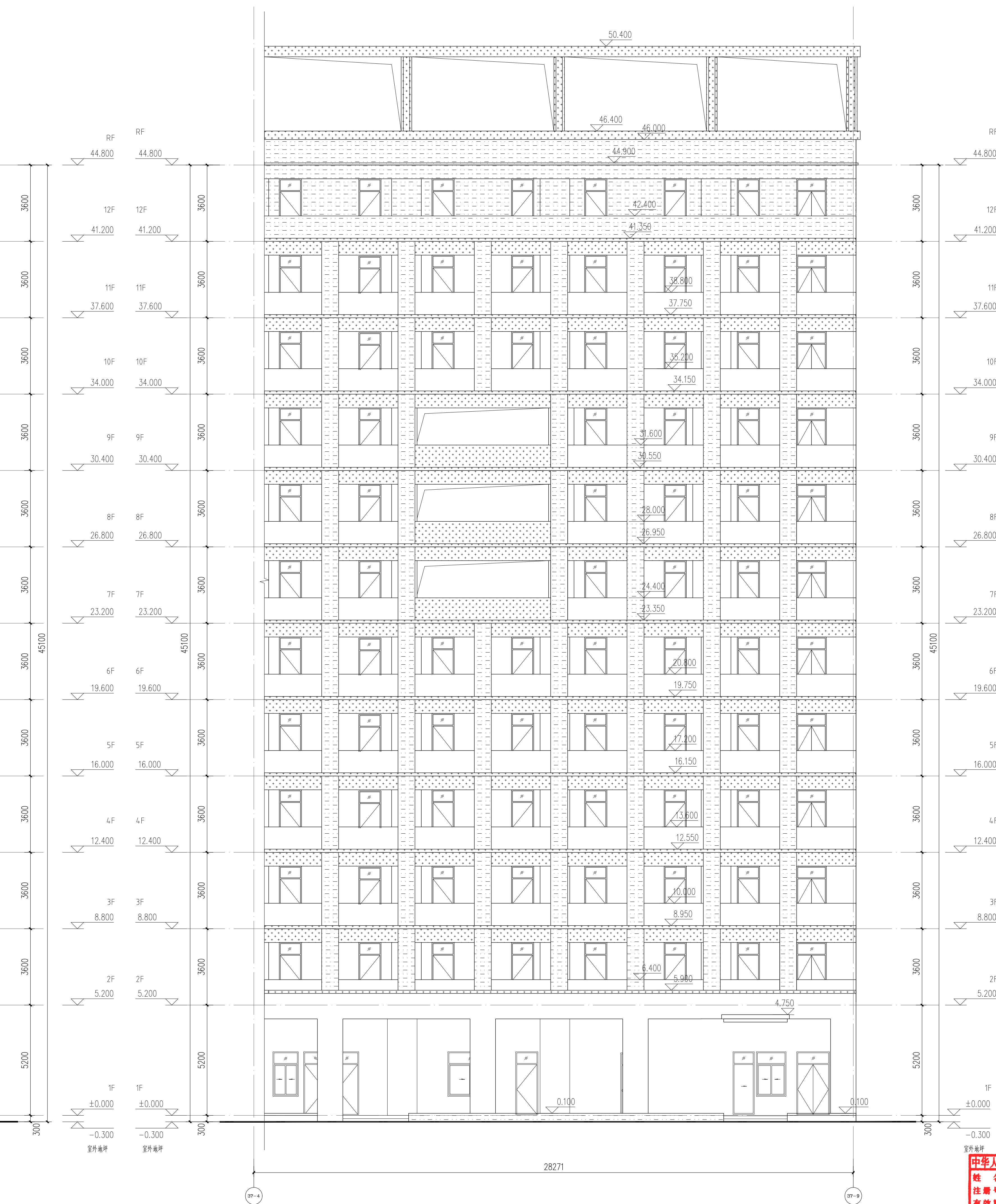
⑪-4~⑪-5 立面图 1:100
