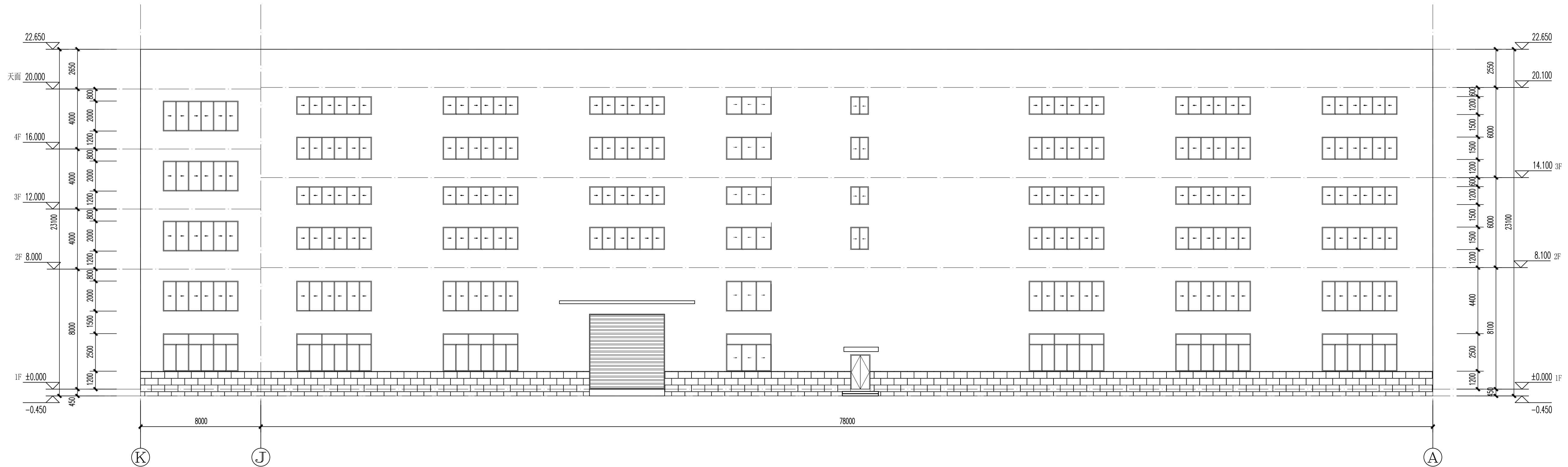
K-A剖面图 1:150
