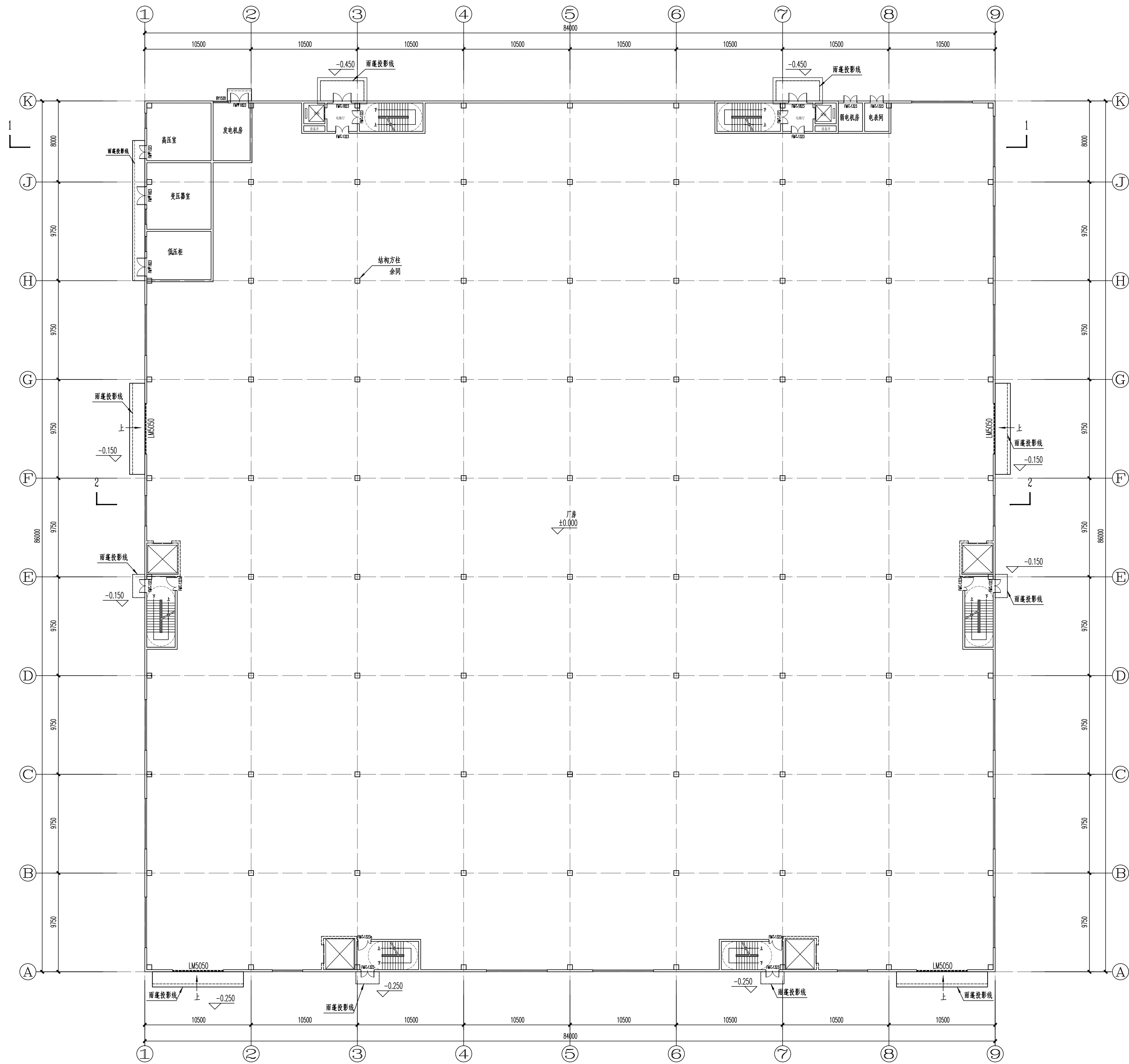
首层平面图 1:200
