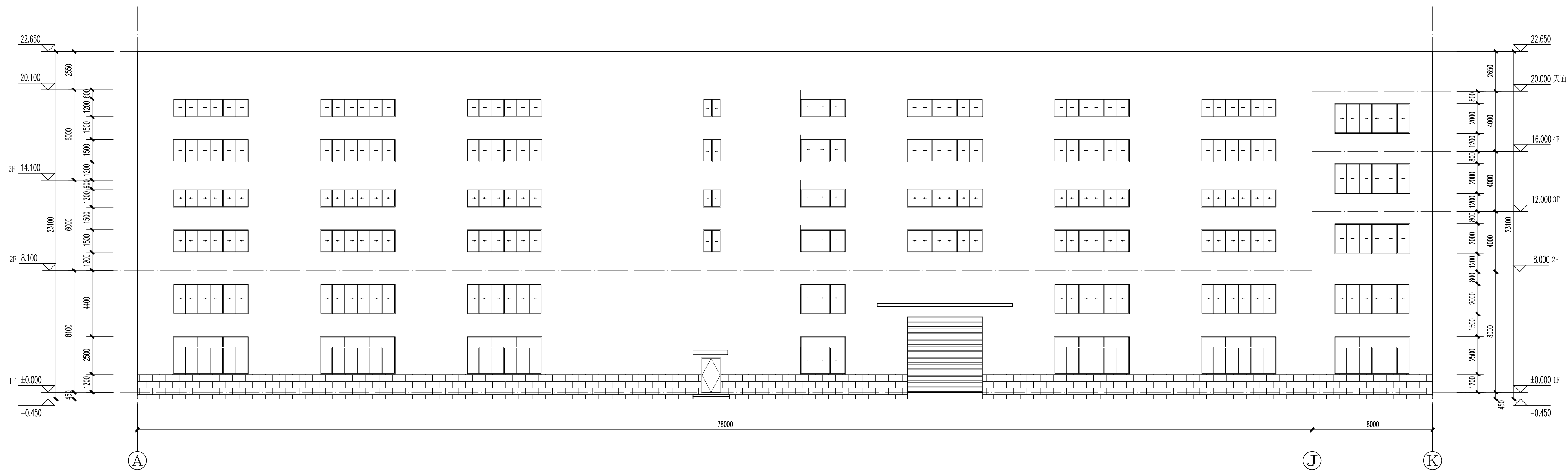
A-K剖面图 1:150
