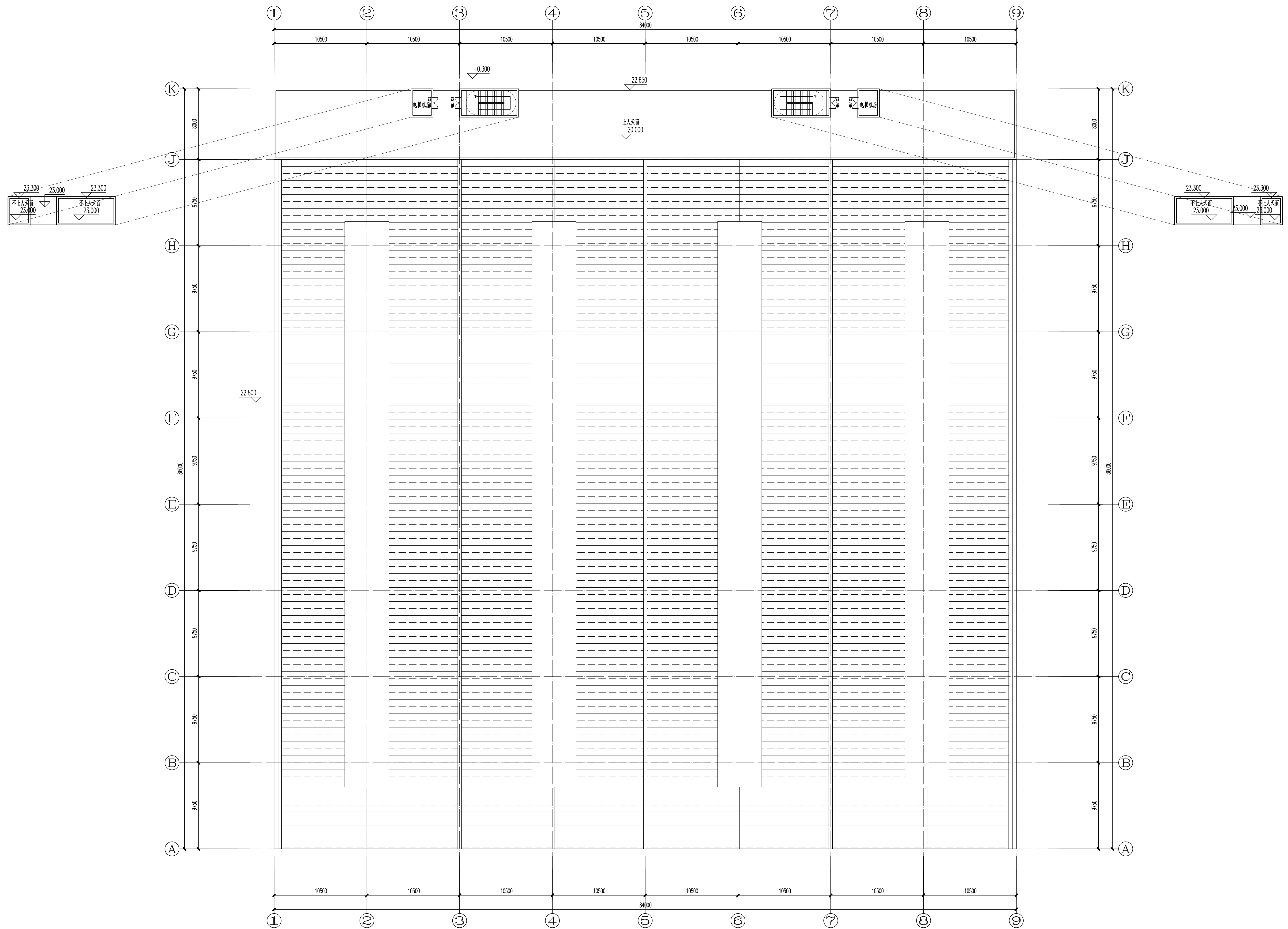
天面层平面图 1:200 本层建筑面积: 58.79平方米 本层计容面积: 0.00平方米
