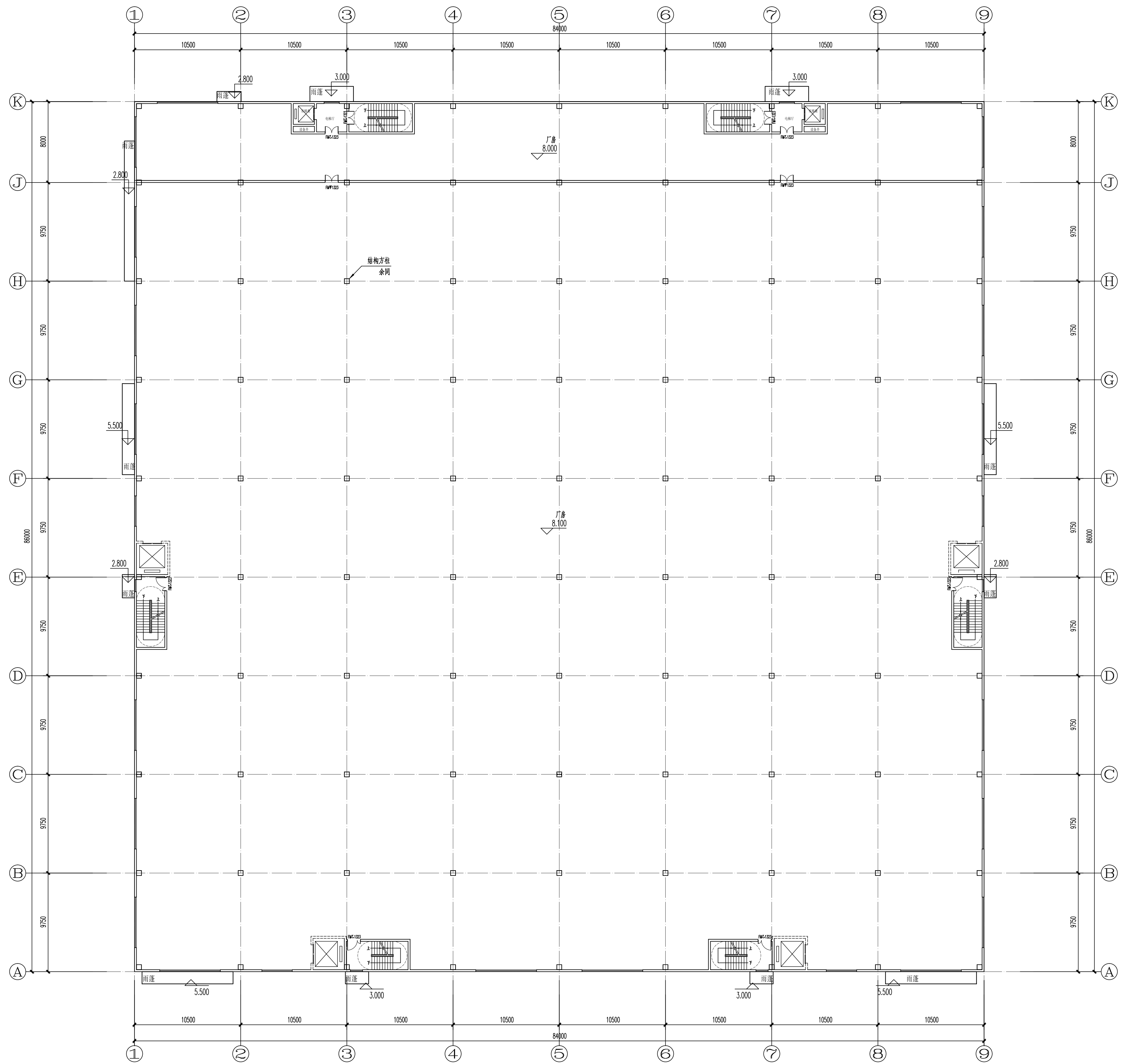
二层平面图 1:200 本层建筑面积: 7224.00 平方米 本层计容面积: 7224.00 平方米
