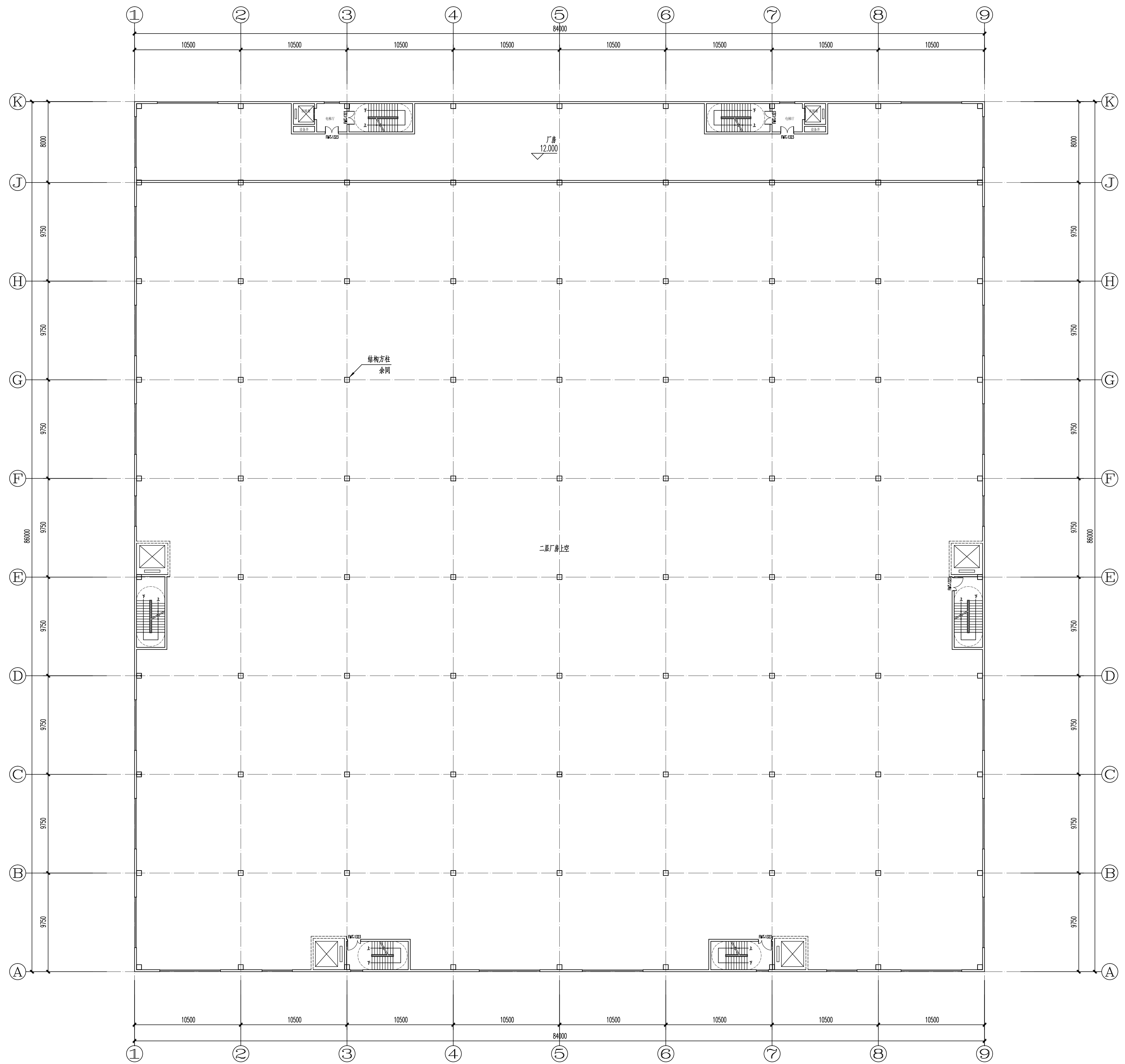
三层平面图 1:200 本层建筑面积: 655.20平方米 本层计容面积: 655.20平方米
