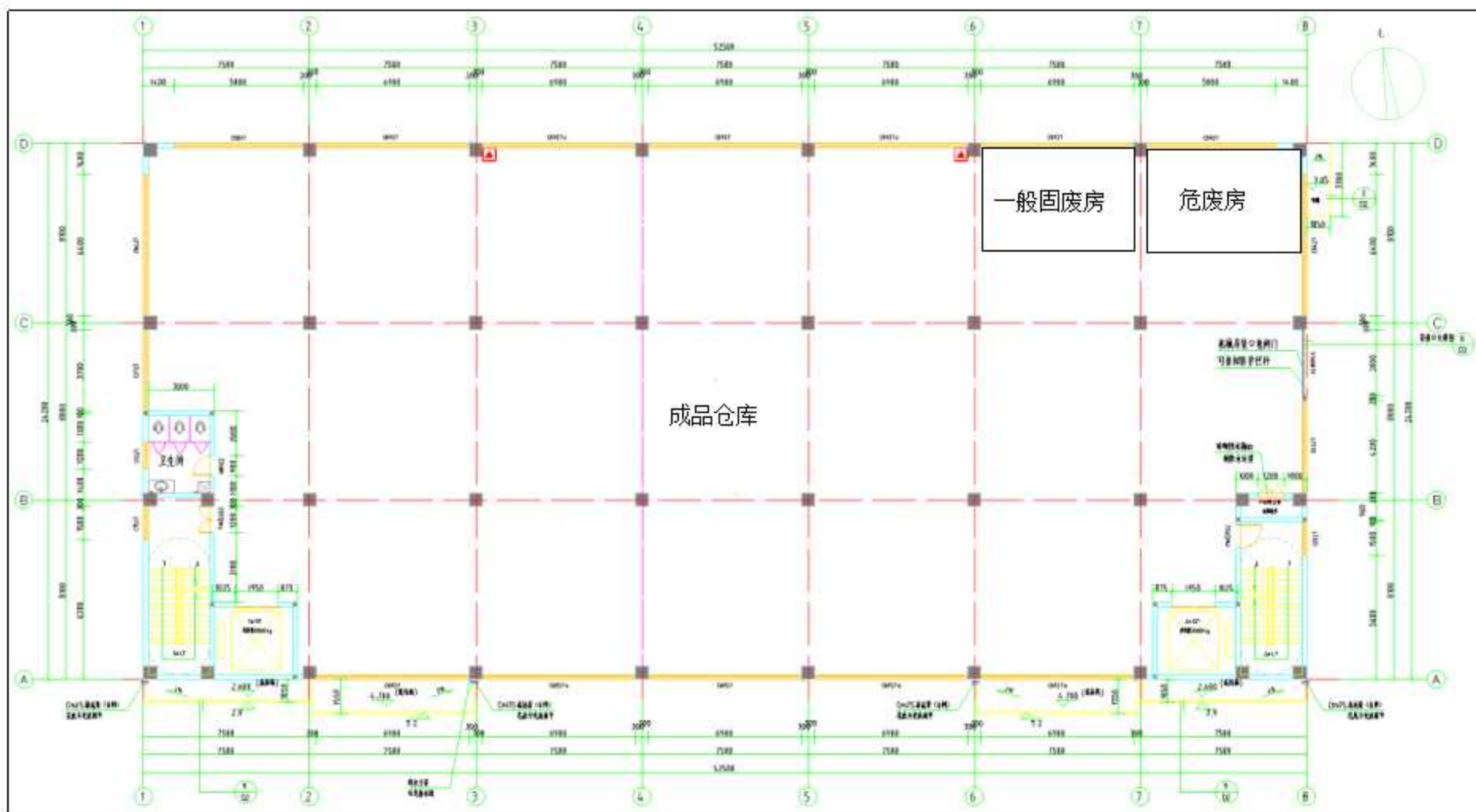
附图 8 项目五楼平面布置
