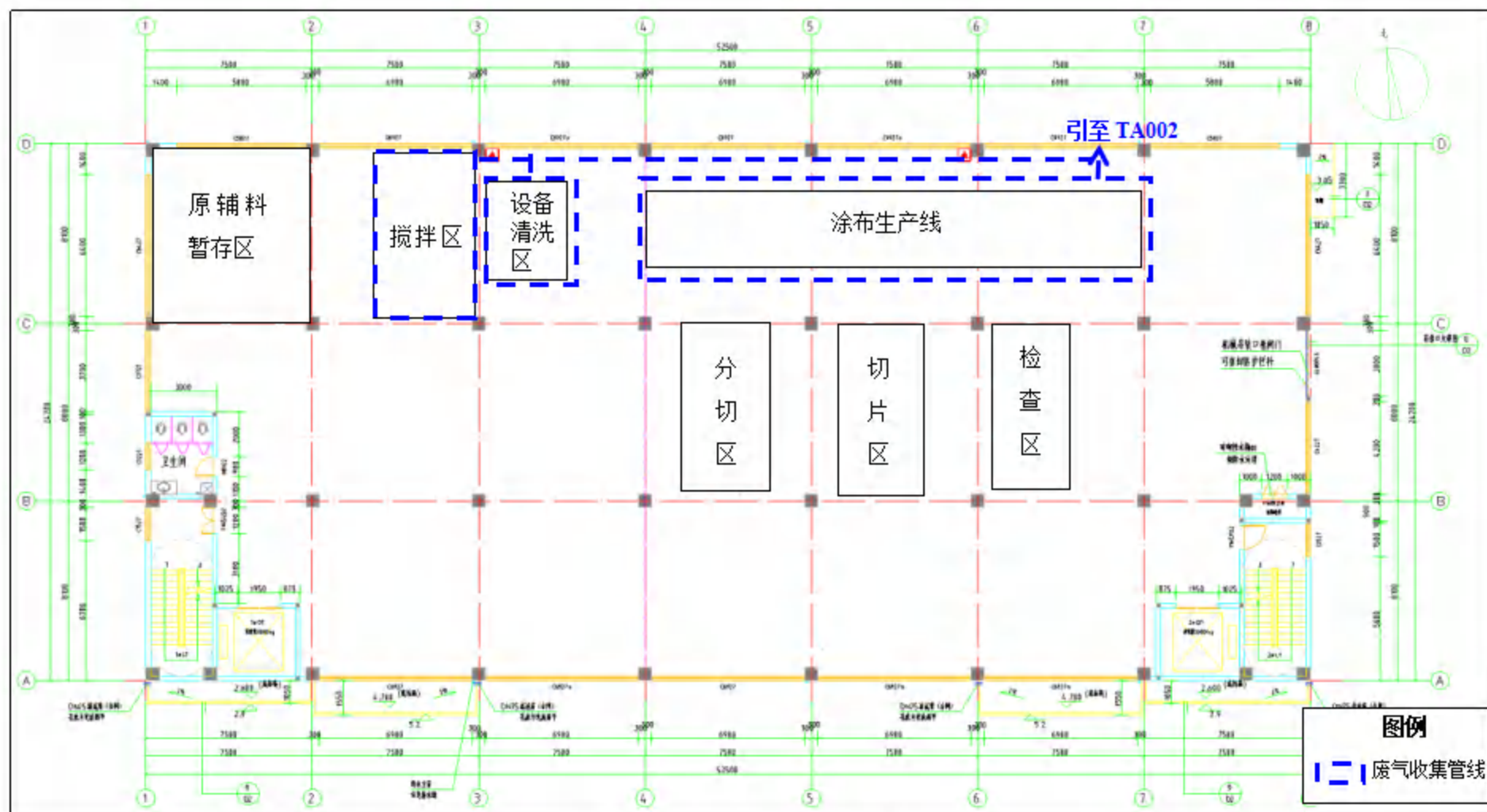
附图 5 项目二楼平面布置图
