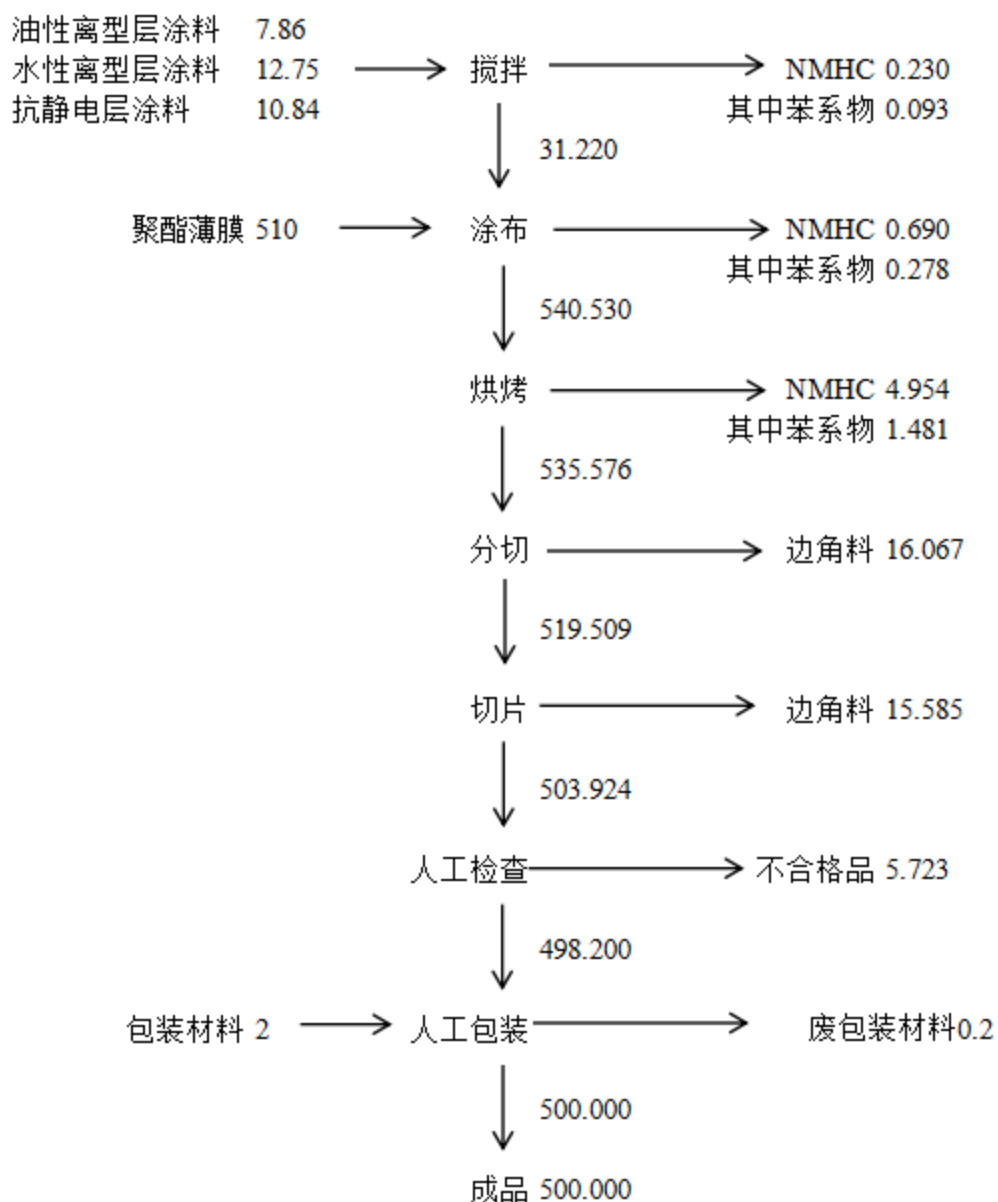
图 2-2 项目物料平衡图 (t/a)
