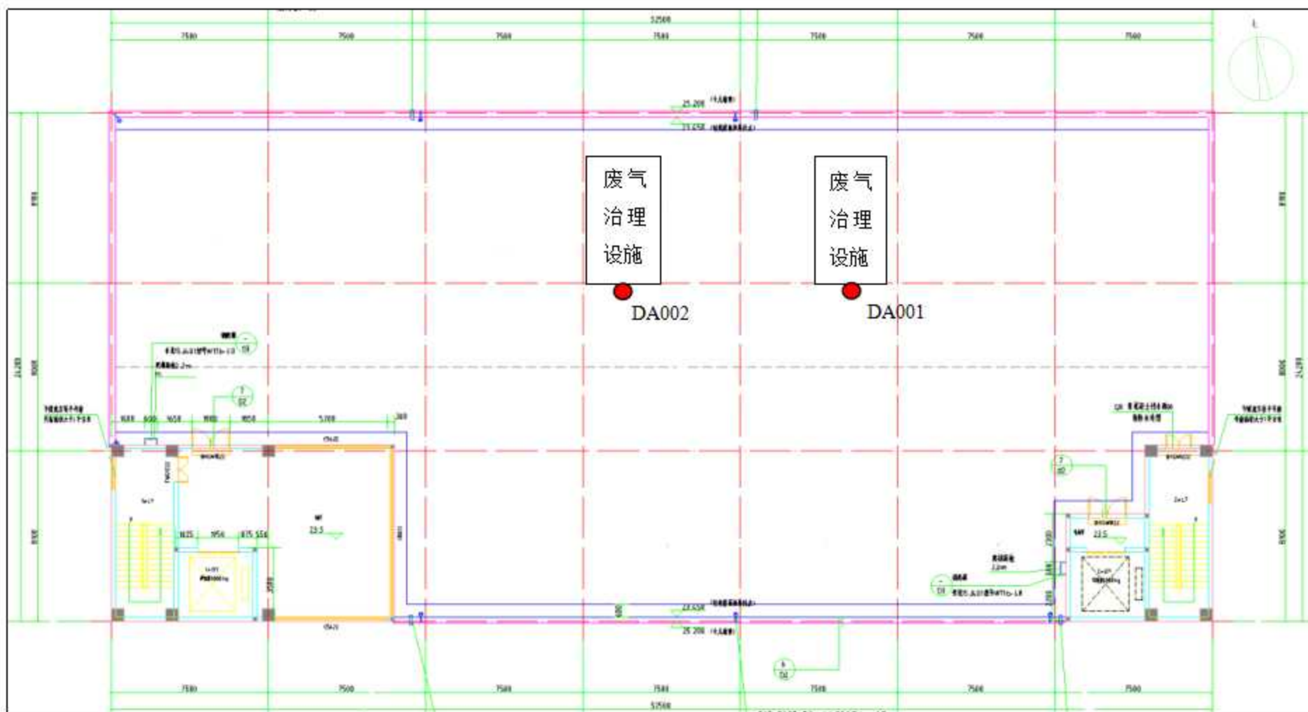
附图 9 项目楼顶平面布置
