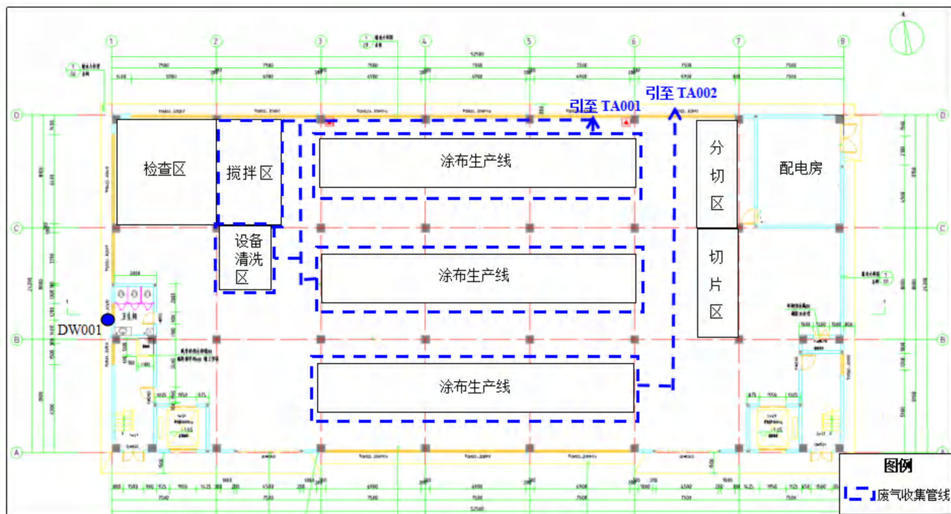
附图 4 项目一楼平面布置图
