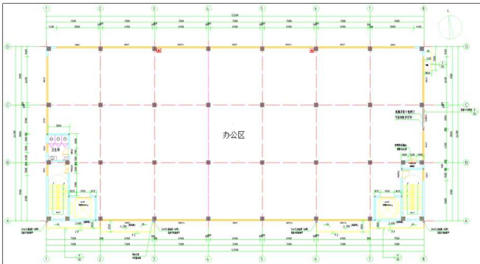
附图 6 项目三楼平面布置图
