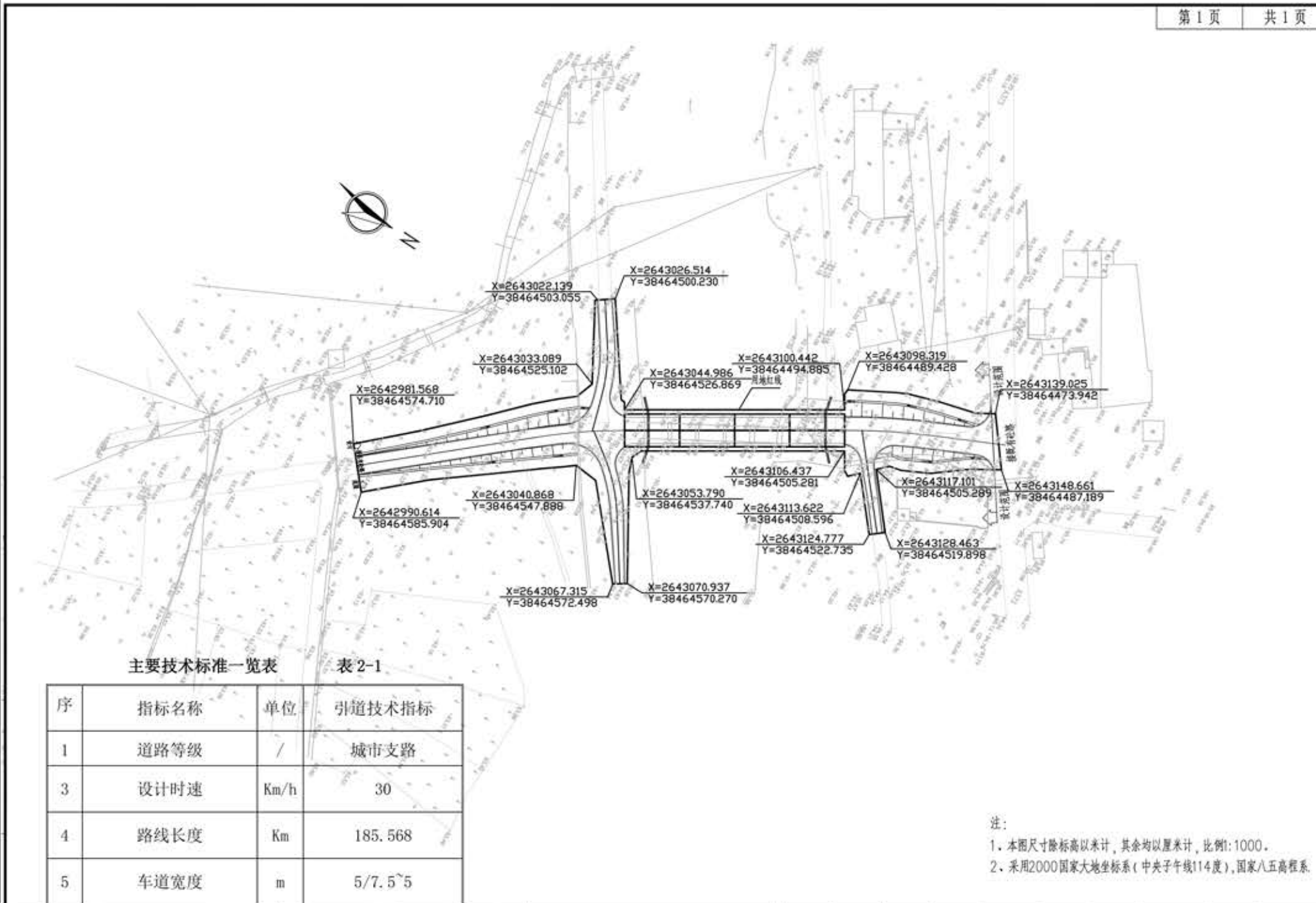
丰二桥 规划总平面图
